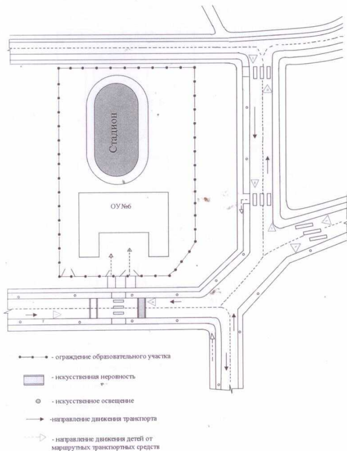
Схема организации дорожного движения в непосредственной близости от образовательного учреждения с размещением соответствующих технических средств, маршруты движения детей
